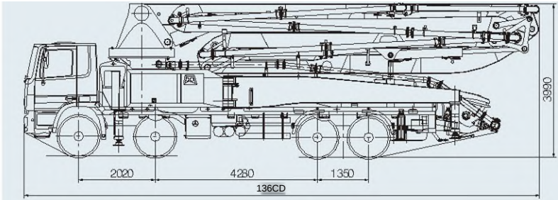
Dimensions
