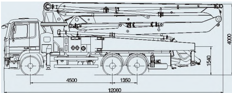
Dimensions
