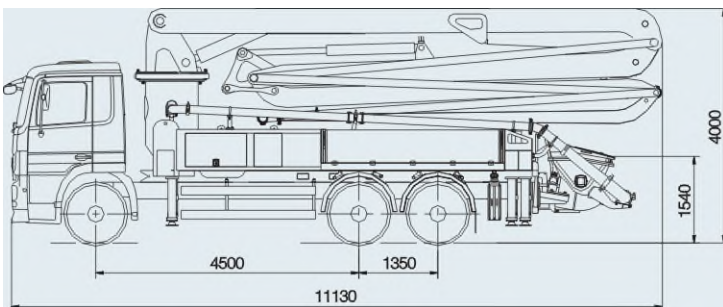
Dimensions
